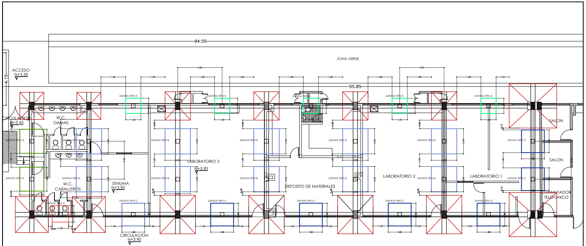
REFORZAMIENTO ESTRUCTURAL EDIFICIO DE LABORATORIOS FACULTAD DE CIENCIAS NATURALES, EXACTAS Y DE LA EDUCACION
